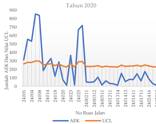
Gambar 3. Hasil Penentuan LRK Prioritas Tahun 2020
